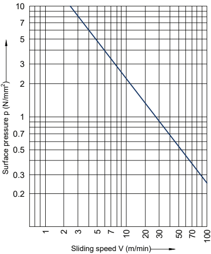
Fig.1 pV value
